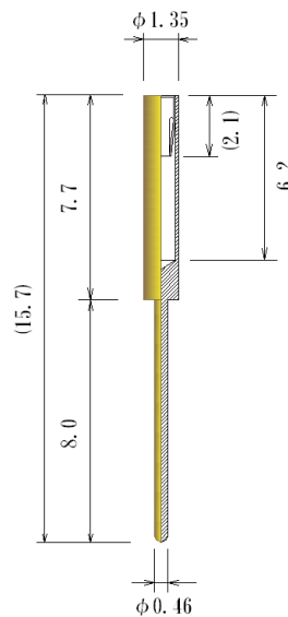
JS135KM-GG
