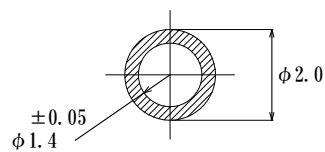
JSS17-GG
