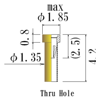
JSP0020-GG (スリーブ 金メッキ) JSP0020-SN (スリーブ スズメッキ)
