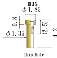
JSP0020-GG (スリーブ 金メッキ) JSP0020-SN (スリーブ スズメッキ)
