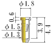
J021-GG
