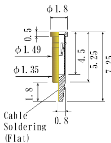
JSC0030-GG
